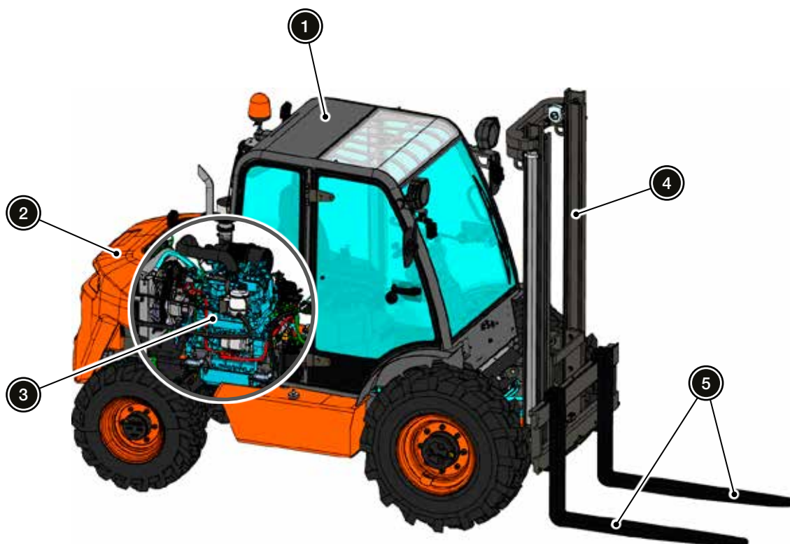
Elementos de la máquina
