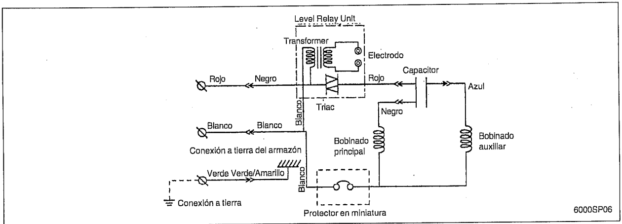
FIGURA 1.6 FUENTE DE PODER LB-480A DE UNA SOLA FASE
