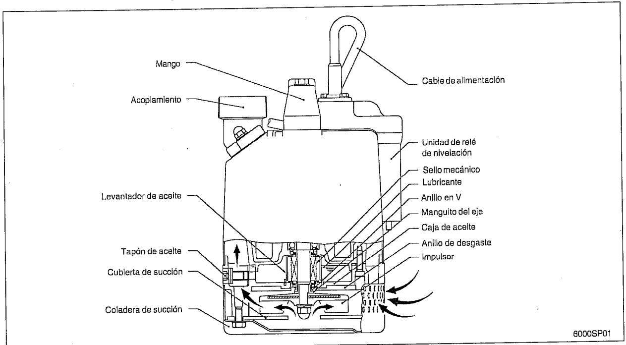
FIGURA 1.1 LISTA DE PARTES
