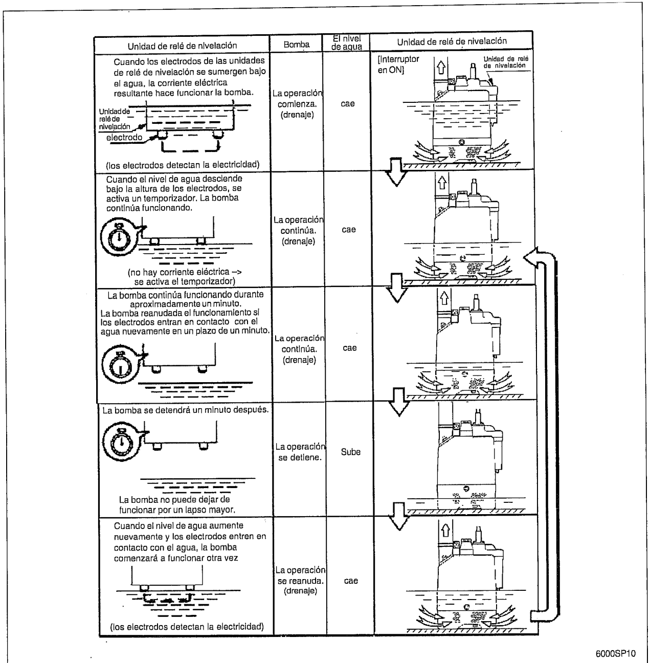
FIGURA 1.10 MANEJANDO EL CICLO DE TIPO AUTOMÁTICO (LB-480A)
