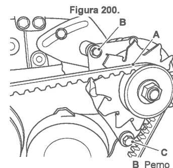
A Correa del ventilador C Perno
