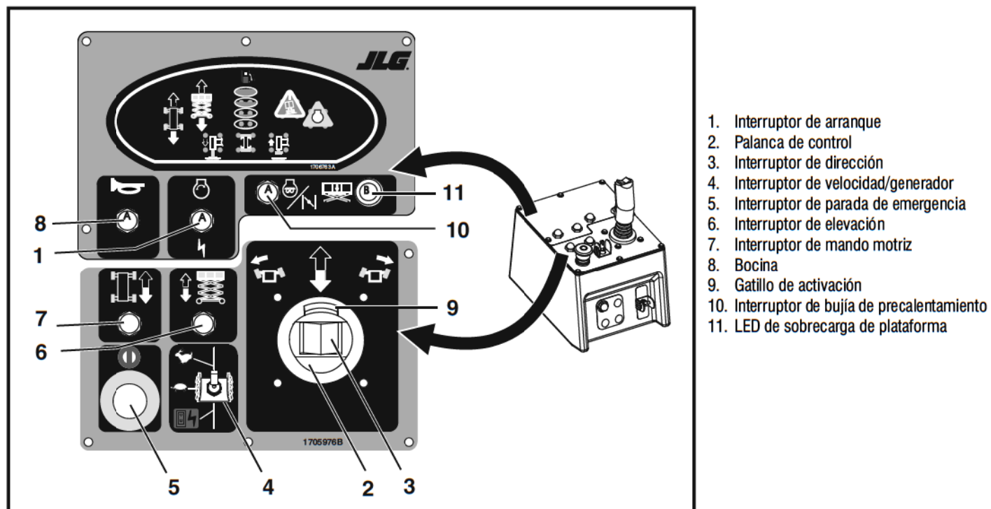
Figura 3-2. Puesto de controles de plataforma
