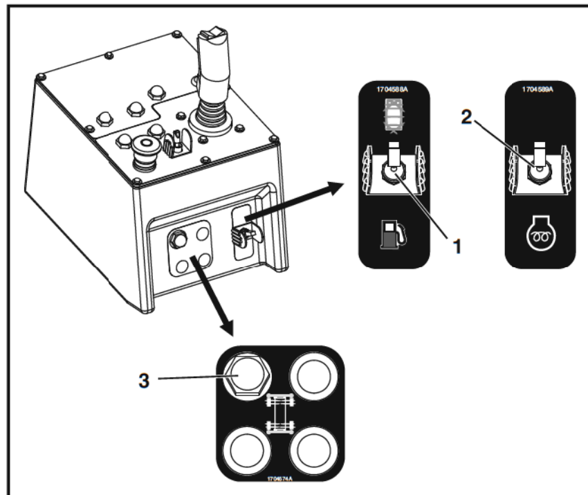
Figura 3-3. Tablero frontal de control de plataforma
