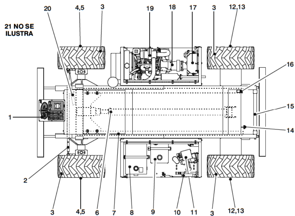
Figura 2-1. Diagrama de inspección visual diaria
