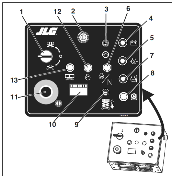
Figura 3-1. Puesto de controles de suelo
