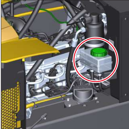
Fig. 213: Posición del depósito del líquido de frenos
