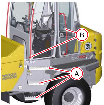
Fig. 72: Subir y bajar, cabina
