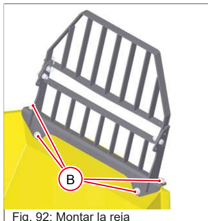
Fig. 92: Montar la rejilla
