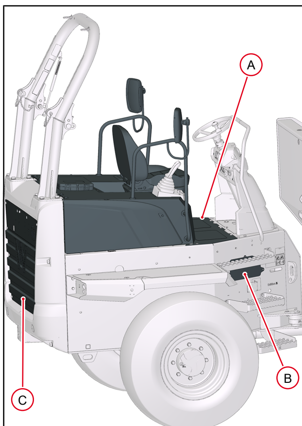
Fig. 183: Accesos de mantenimiento, barra antivuelco
