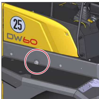
Fig. 200: Controlar el nivel de aceite hidráulico
