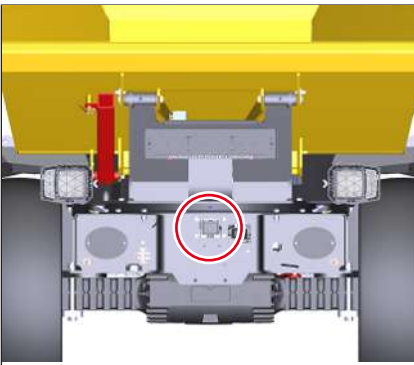
Fig. 118: Sensor ASC volquete
