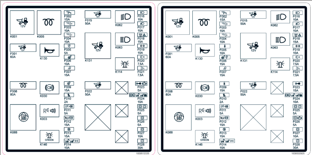
Fig. 240: sin ASC/con ASC
