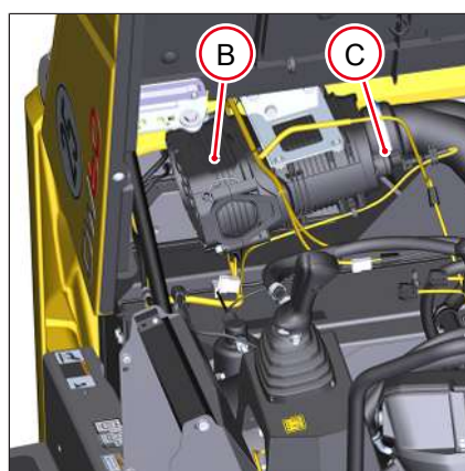
Fig. 226: Aspiración de aire
