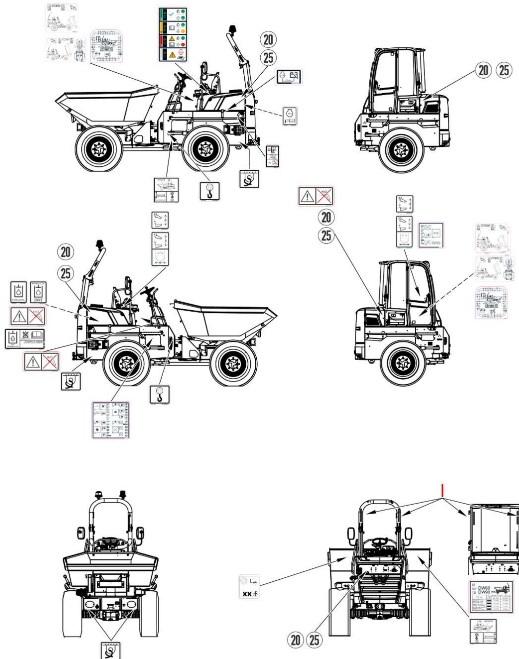
Fig. 27: Vista general de los adhesivos de indicaciones
