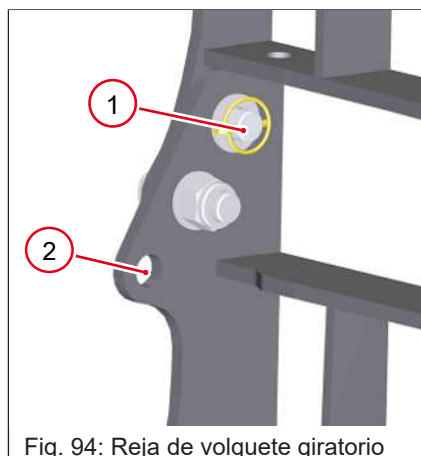
Fig. 94: Reja de volquete giratorio
