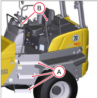
Fig. 71: Subir y bajar, barra antivuelco
