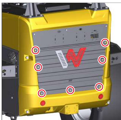
Fig. 229: Rejilla de ventilación (representación simbólica)
