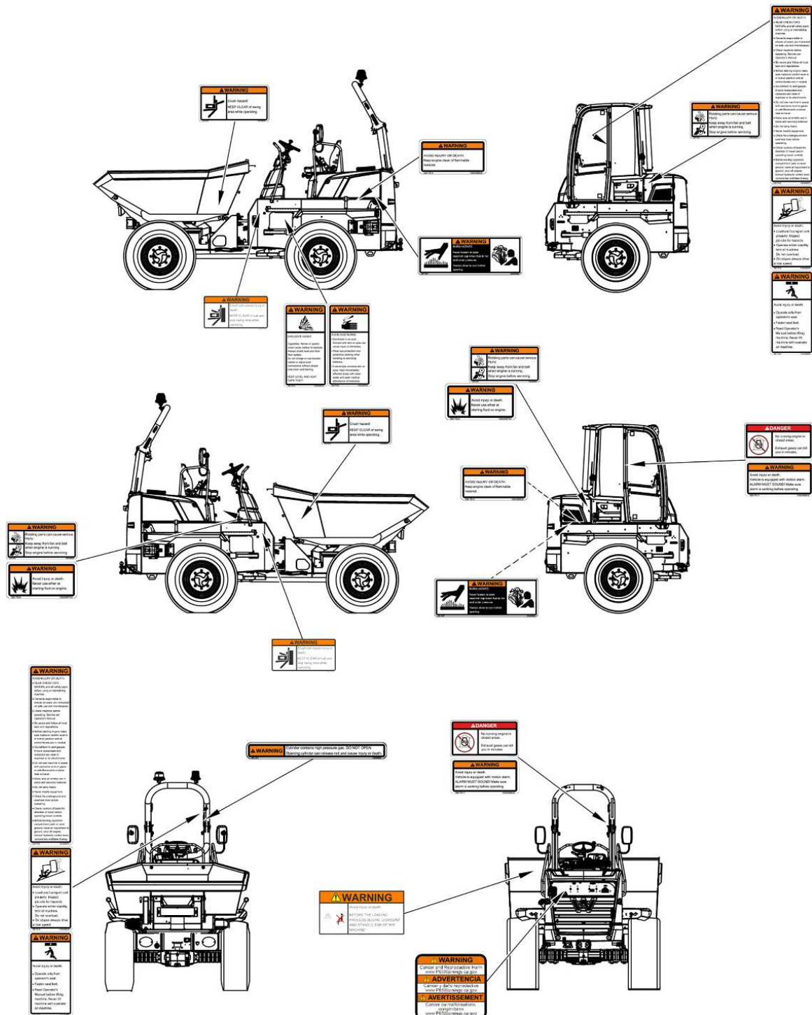
Fig. 54: Vista general de adhesivos ANSI
