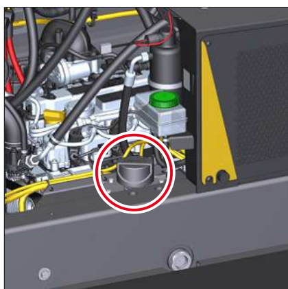
Fig. 201: Abertura de llenado de aceite hidráulico
