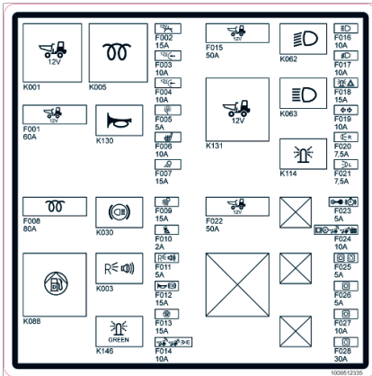
Fig. 49: Adhesivo: fusibles (representación simbólica)
