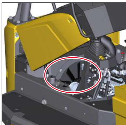
Fig. 228: Parte interior de la carcasa del ventilador
