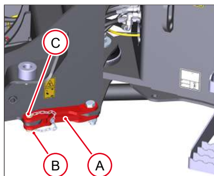
Fig. 174: Bloqueo articulado desmontado
