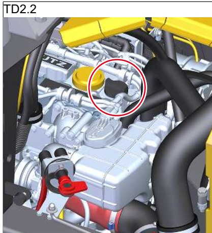
Fig. 208: Abertura de llenado para el aceite del motor
