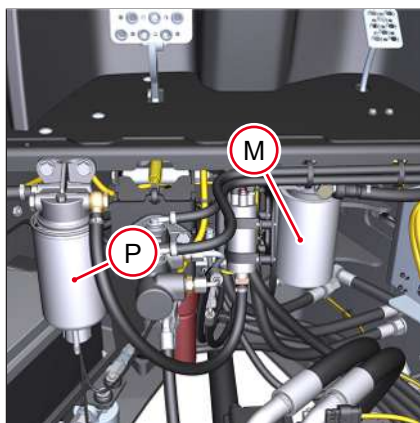
Fig. 203: Filtro de combustible
