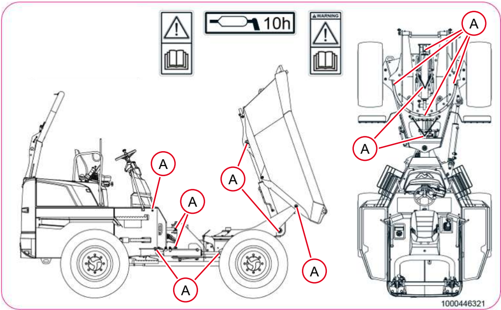
Fig. 224: Programa de lubricación volquete giratorio
