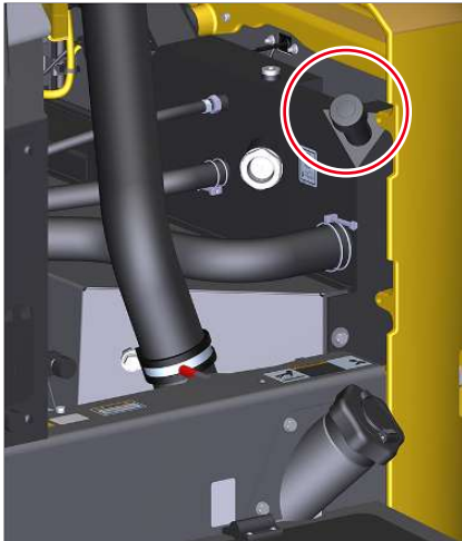
Fig. 212: Abertura de llenado para el agente refrigerante
