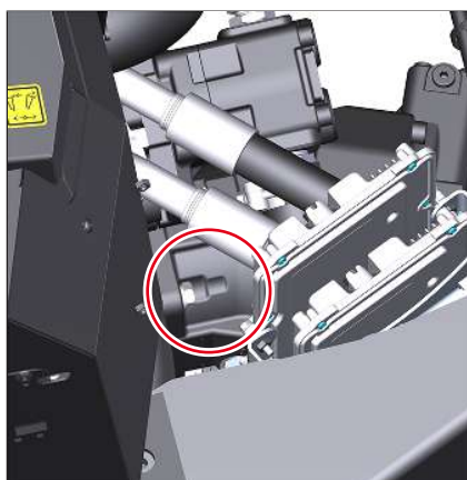
Fig. 169: Válvula derecha limitadora de presión
