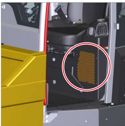
Fig. 189: Filtro grueso
