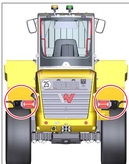
Fig. 144: Luces traseras y de gálibo
