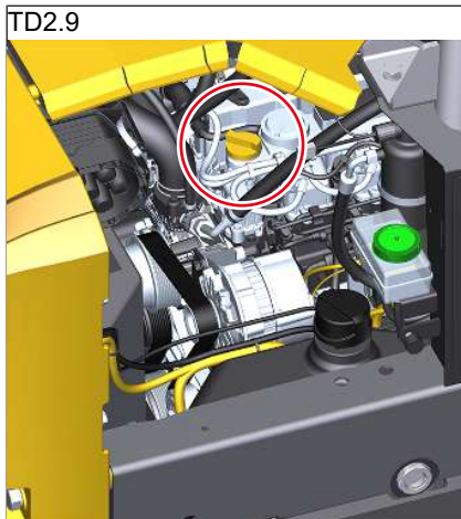
Fig. 209: Abertura de llenado para el aceite del motor
