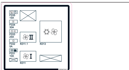
Fig. 50: Adhesivo: fusibles (representación simbólica)
