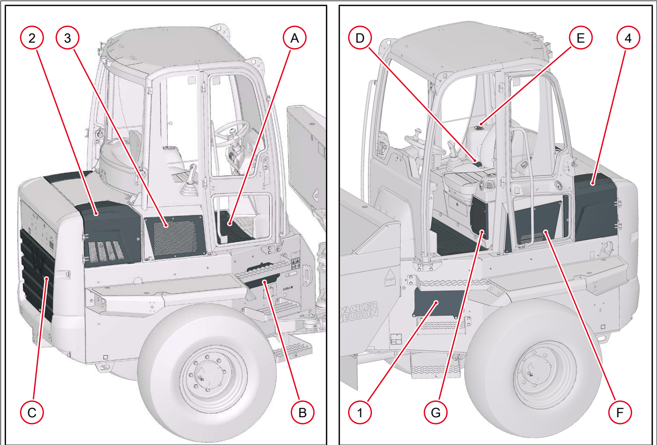
Fig. 184: Accesos de mantenimiento cabina
